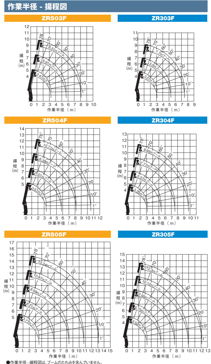
●作業半径・揚程図は、ブームのたわみを含んでいません。
