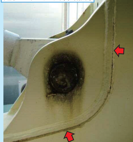
起伏シリンダ下部支点部
